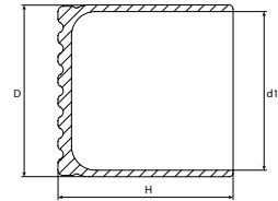
KESİT A-A
