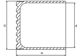
KESİT A-A
